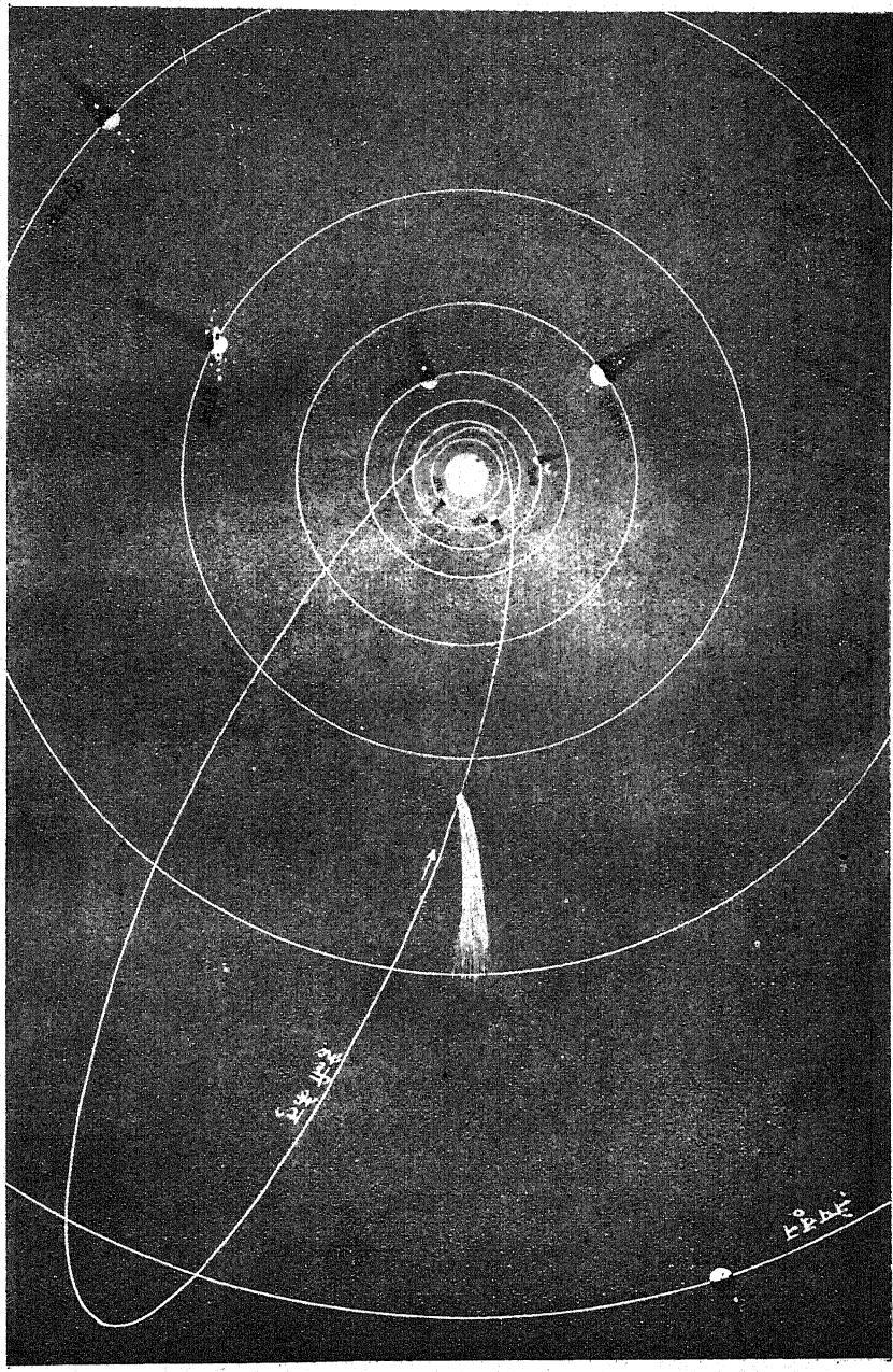
चित्र २२—सौर परिवार । इसमें डेढ़ हज़ार के लगभग नरहें-नरहें अवतार ग्रह भी हैं, जो दिखाये नहीं जा सके हैं । सौर-परिवार से
